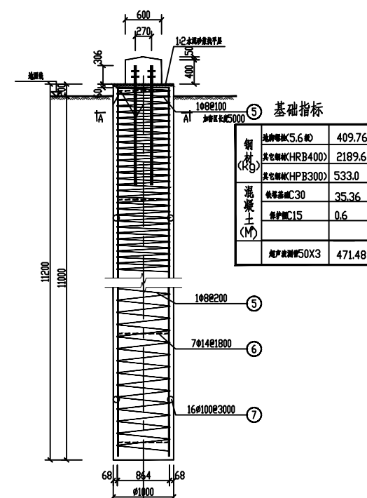
35-CD22S-J2灌注桩基础
