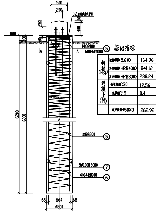
35-CD22S-Z2灌注桩基础
