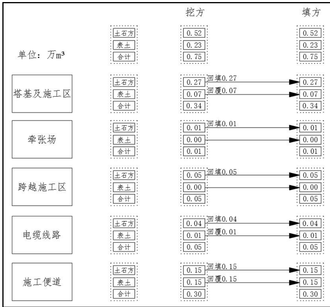
图 2-5 总土石方流向框图
